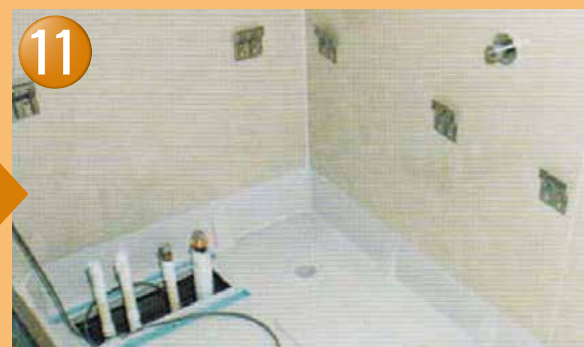
バス組立て
